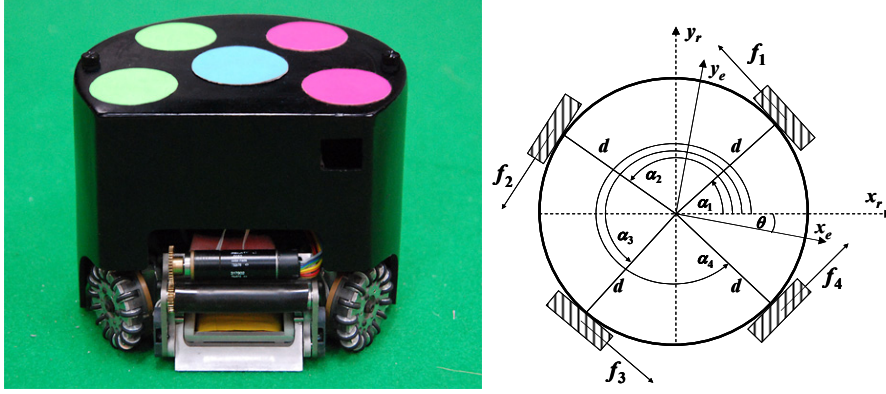
Fig. 2. Skuba 2009 robot
